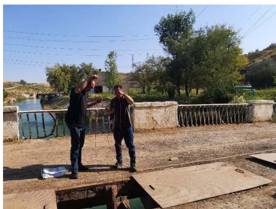
Фото: Замеры расхода воды и электроэнергии на насосной станции ГНС-1 при поддержке Grundfos
